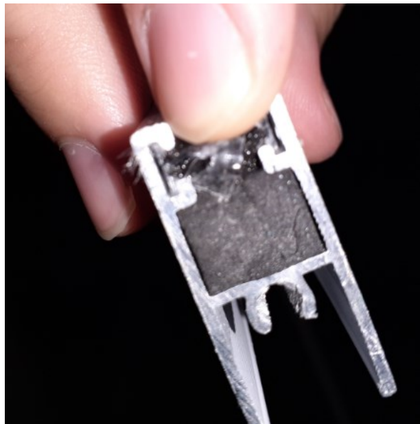
Foto 8 – Manta de composto plástico que preenche as travessas superior e inferior da folha.
