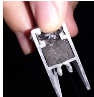
Foto 9 – Manta de composto plástico que preenche as travessas superior e inferior da folha
